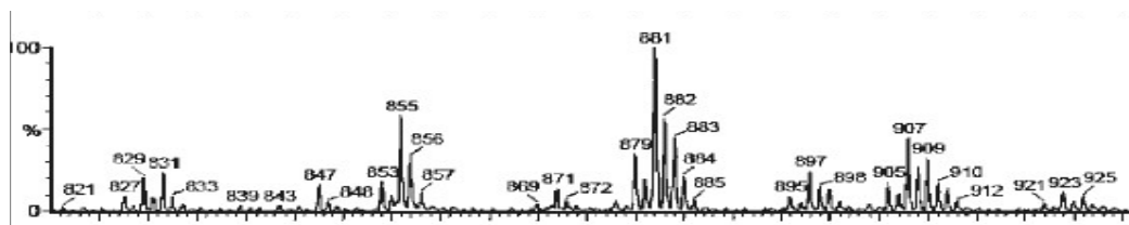
Figura 7 – Fragmentos de massa do óleo de andiroba obtido por meio da técnica de espectrometria de massa (MALDI-TOF MS) 88
