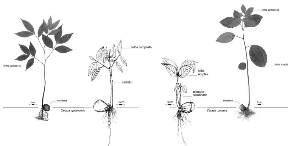
Figura 5 – Representação de plântula das espécies Carapa guianensis Aubl. e Carapa procera D.C. 5
