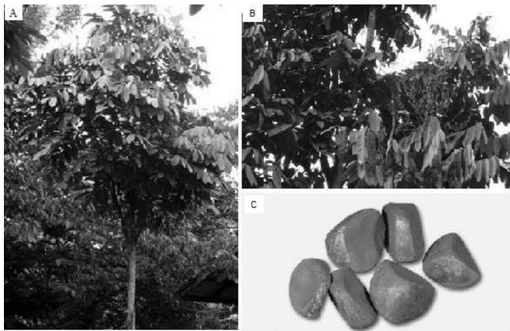
Figura 1 – Indivíduo jovem (A), ramo com folhas e flores (B) e sementes (C) de Carapa guianensis Aubl.
