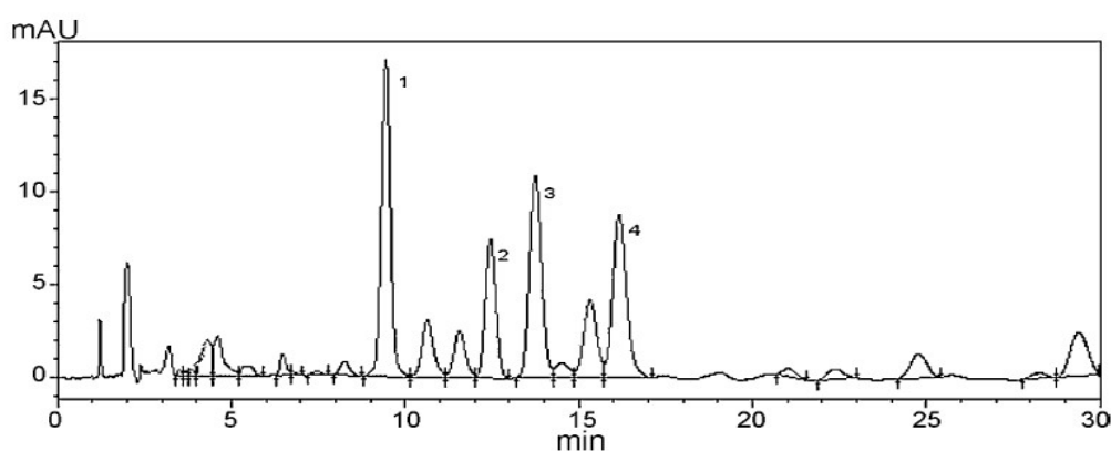
Figura 6 – Perfil cromatográfico do óleo de andiroba obtido por HPLC-PAD indicando a presença de (1) 7-deacetoxi-7-oxo-gedunina, (2) angolensato de metila, (3) 6α-acetoxigedunina e (4) gedunina 23
