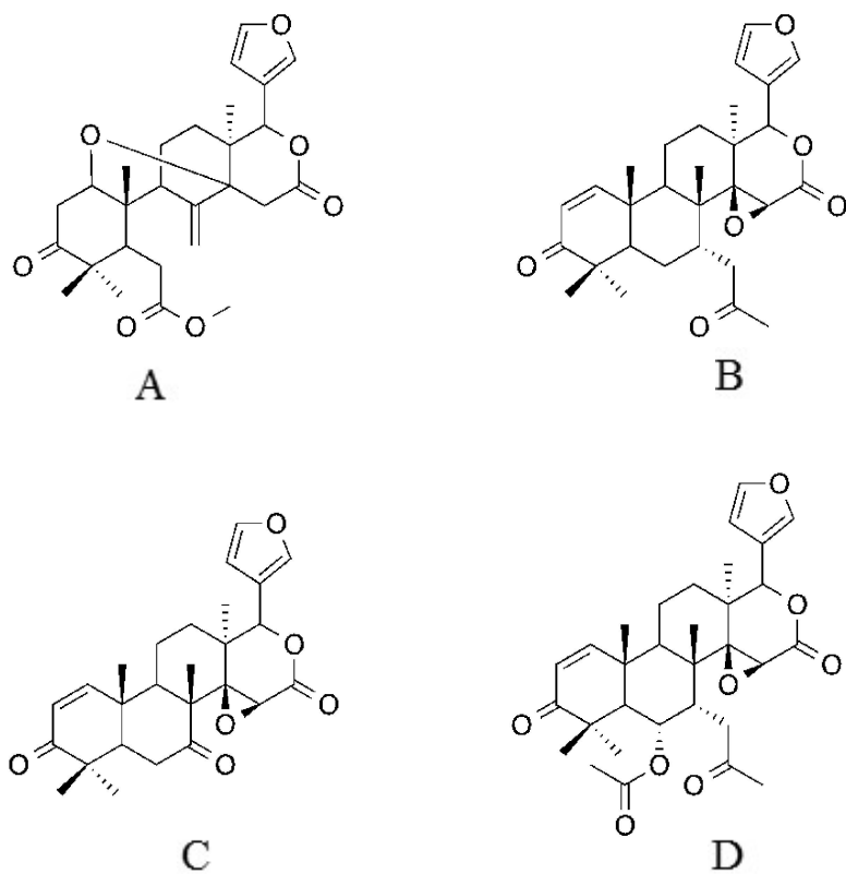
Figura 8 – Principais tetranortriterpenoides que constituem a fração insaponificável do óleo de andiroba: (A) angolensato de metila, (B) gedunina, (C) 7-deacetoxi-7-oxo-gedunina e (D) 6 \alpha -acetoxigedunina 23
